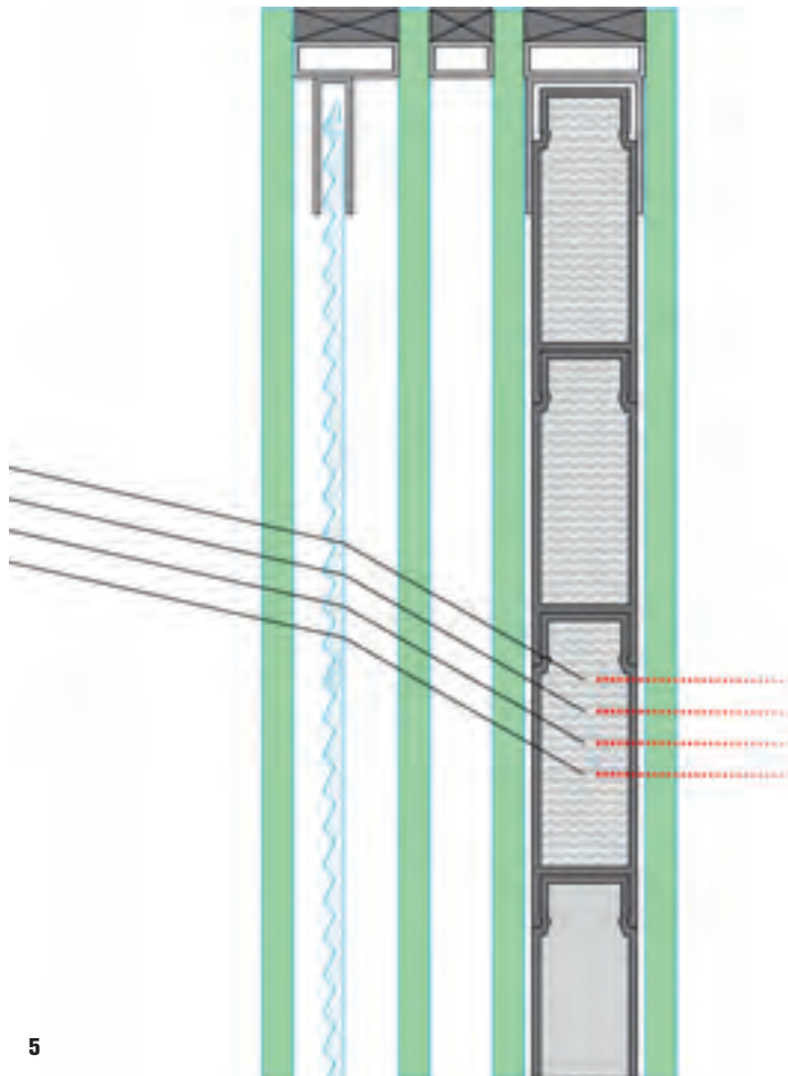
5 Latentspeicherwand von Dietrich Schwarz, Winterzustand 6 + 7 Alterswohnungen in Domat/ Ems, Dietrich Schwarz, 2004 (Bilder: Dietrich Schwarz) 8 Hautausschnitt (www.biologie.de)
